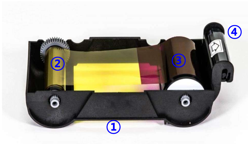
Figure 7 Характеристики съёмного картриджа для лент
