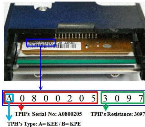
Рис. 111 Термопечатная головка
