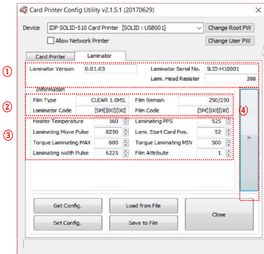
Рис. 10 CardPrinterConfig – базовые настройки ламинатора
